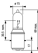
M5 (BA20d)
