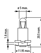
Bax EBS-R
