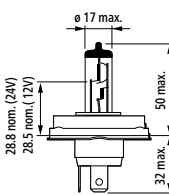
R2 Halogen
