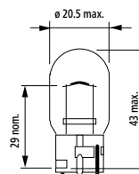
W(Y)21W
