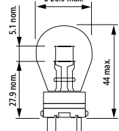
3157
