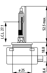
D1R
