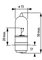
M5 (P15d-25-1)
