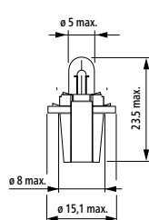
Bax 8,3d
