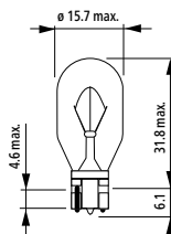
W16W
