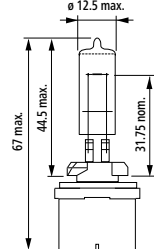
885, 893
