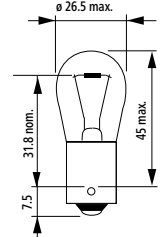
P(Y)21W
