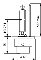
D2S, D4S
