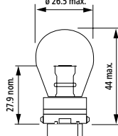
3156
