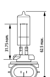
886, 894, 896
